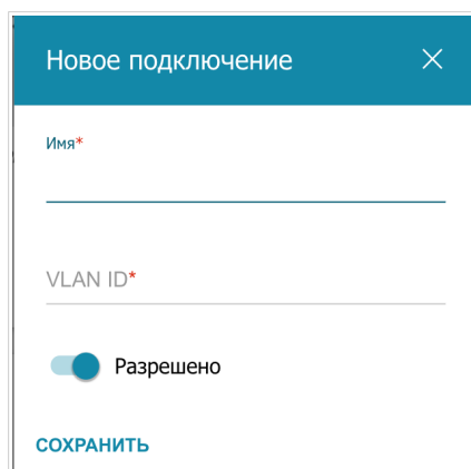
Рисунок 54. Добавление подключения.
