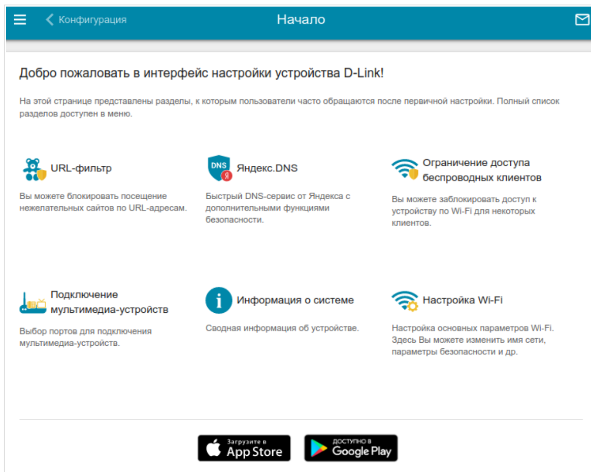
Рисунок 26. Страница Начало .
